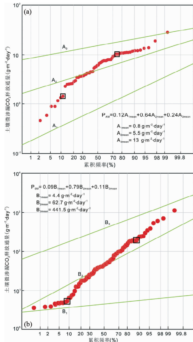
图5 土壤微渗漏 CO 2 释放通量的对数累积频率分布图 (a)-三条绿色直线分别为 A 区三组子样本 A 1 、A 2 、A 3 释放通量的平均累积频率曲线; (b)- 三条绿色直线分别为 B 区三组子样本 B 1 、B 2 、B 3 释放通量的平均累积频率曲线. 方框内的点为拐点
