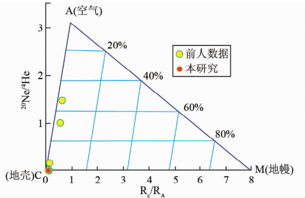
图 6 ^{20}\text{Ne}/^4\text{He} 与 R_C/R_A 相关图 (底图据 Lan et al. , 2007)
