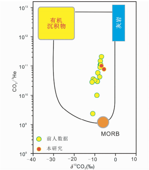
图 8 \text{CO}_2/^3\text{He} 与 \delta^{13}\text{C} 相关图解 (底图据 Lan et al. , 2007)
